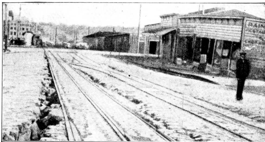
II: Fig. II. — Sprickor i Valentia Street, S. Francisco efter jordbäfningsen år 1906.
