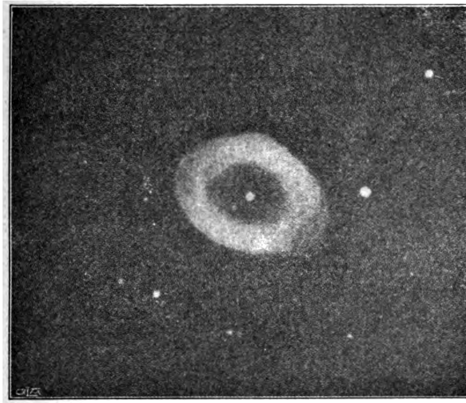
4I: Fig. 4I. — Ringnebulosan i Lyran enligt fotografi från Yerkes-observatoriet.
