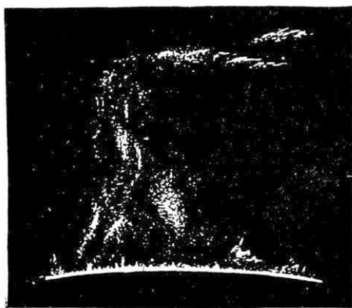
2I: Fig. 2I. — Rökpelarformad lugn protuberans.
