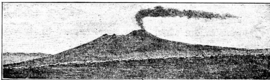
I: Fig. 1. — Vesuvius, sedd från ön Nisita under måttlig vulkanisk verksamhet.
