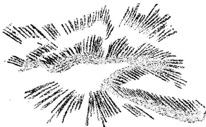
35: Fig. 35. — Norrskens-korona observerad på Spetsbergen 1883.
