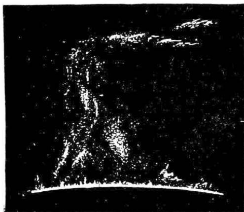
21: Fig. 21. — Rökpelarformad lugn protuberans.
