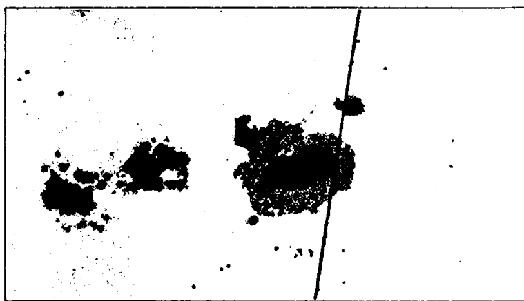
17: Fig. 17. — Samling av solfläckar på solskifvan den 8 Sept. 1898. Strecket på bilden anger läget av solens centrala meridian.
