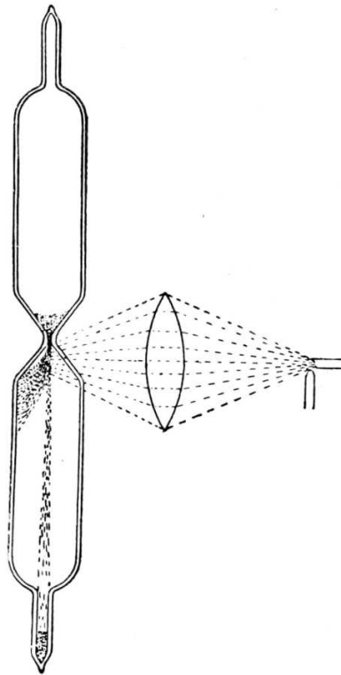
31: Fig. 31. — Nichols och Hulls försök att eftergöra kometsvansar, genom att låta elektriskt båggljus, koncentreradt genom en lins, falla på fint pulver.
