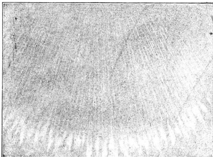
34: Fig. 34. — Norrskensstrålar.
