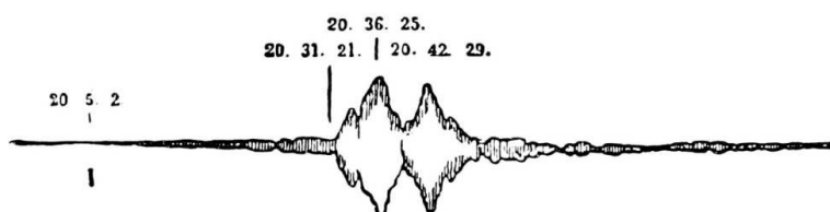
16: Fig. 16. — I Shide upptaget seismogram.
