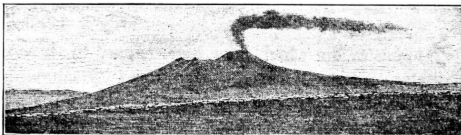
1: Fig. 1. — Vesuvius, sedd från ön Nisita under måttlig vulkanisk verksamhet.
