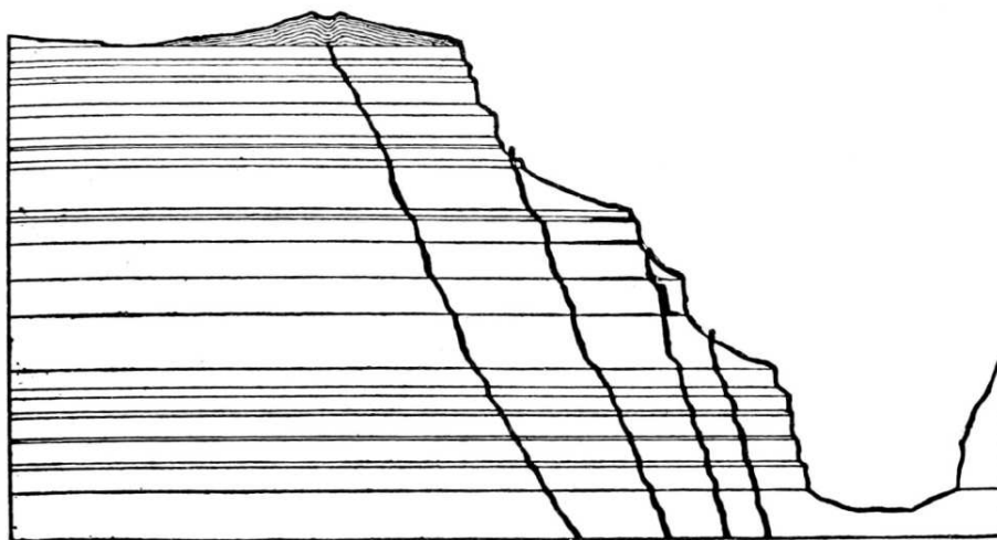
8: Fig. 8. — Lavafyllda sprickor med en vulkanisk askkägla på Torowheap-canon, Colorado-platån. Skematisk bild.
