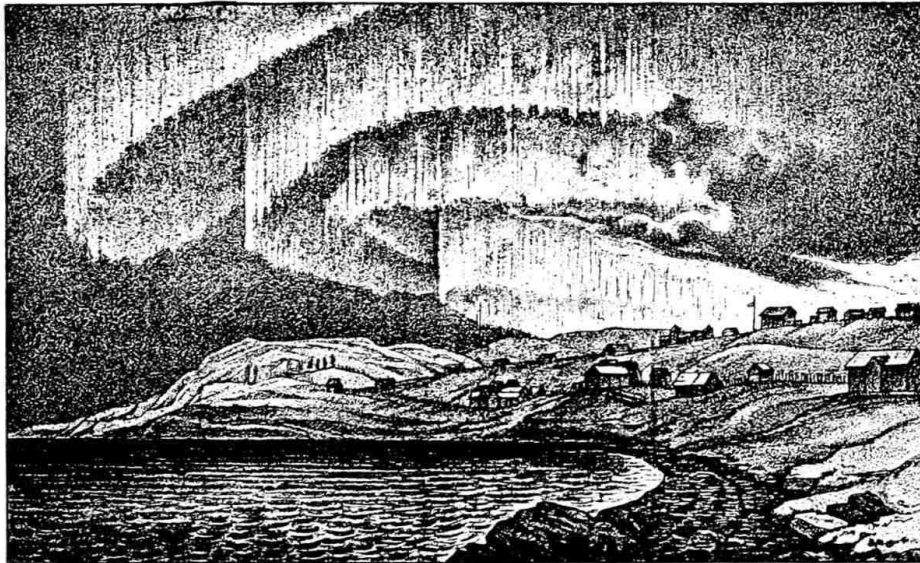
36: Fig. 36. — Draperinorrskenen observeradt i norra Norge.
