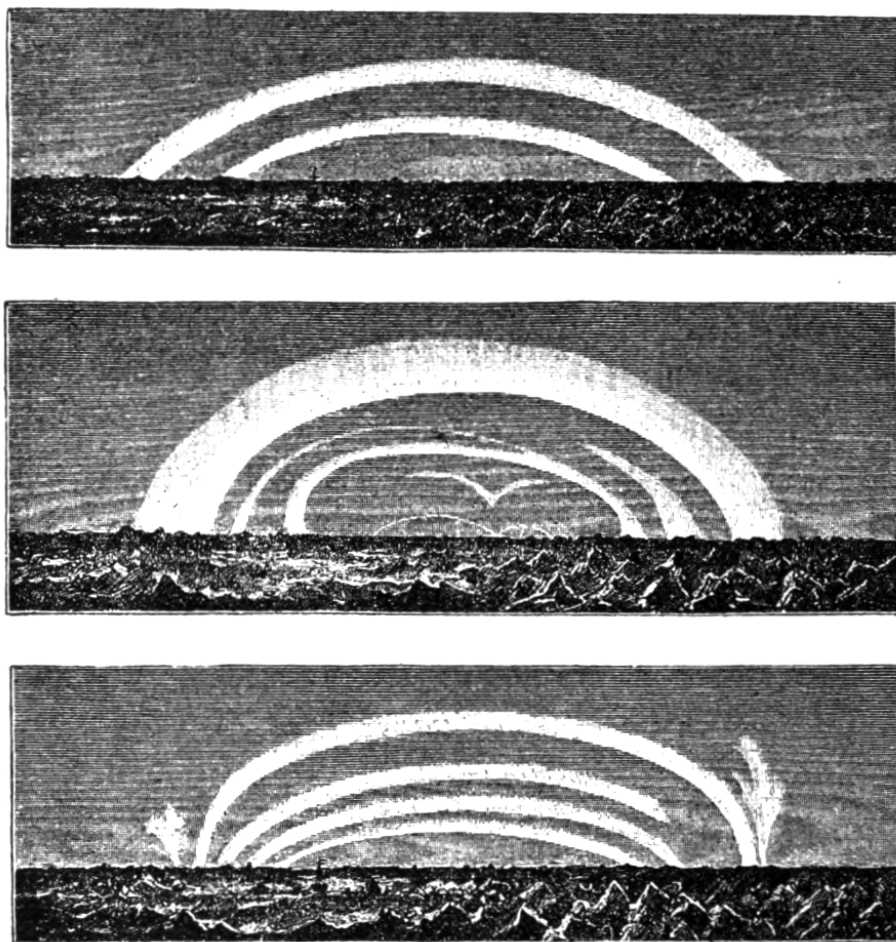
33: Fig. 33. — Bågformade norrsken iakttagna av Nordenskiöld under Vegas övervintring nära Behrings sund 1879-80.
