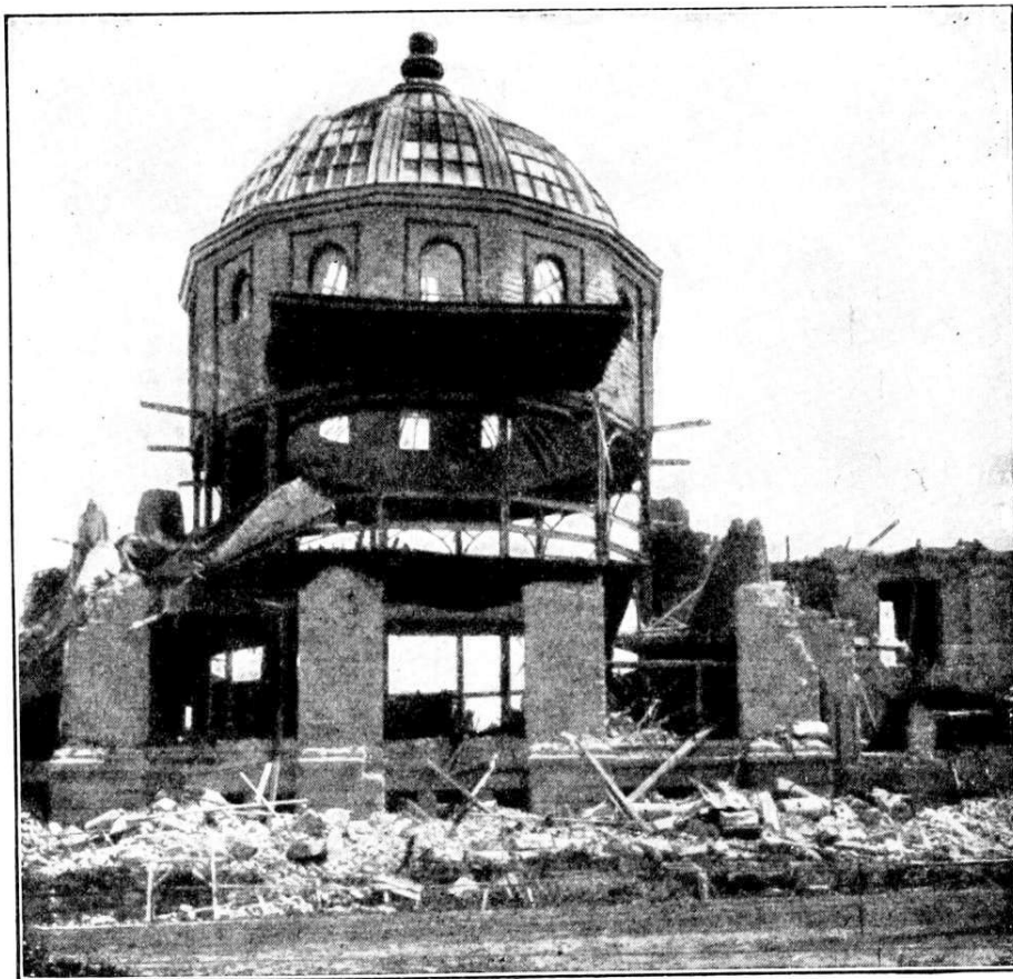
14: Fig. 14. — Universitetsbiblioteket vid Stanford University i Kalifornien efter jordbäfningen 1906. Bilden visar järnkonstruktioners stora hållfasthet, jämförd med murverks. Jordbäfningens inverkan på låga trähus synes på fig. II.
