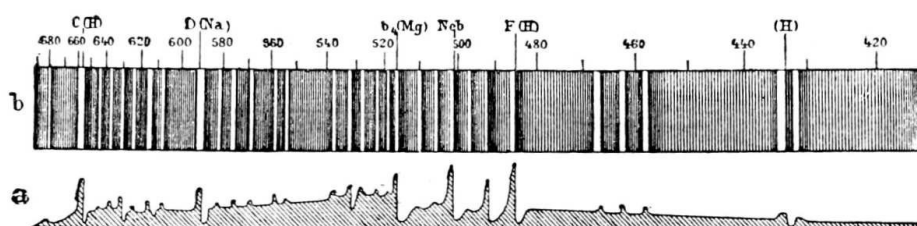
38: Fig. 38. — Spektrum av den nya stjärnan i Kusken av år 1892.
