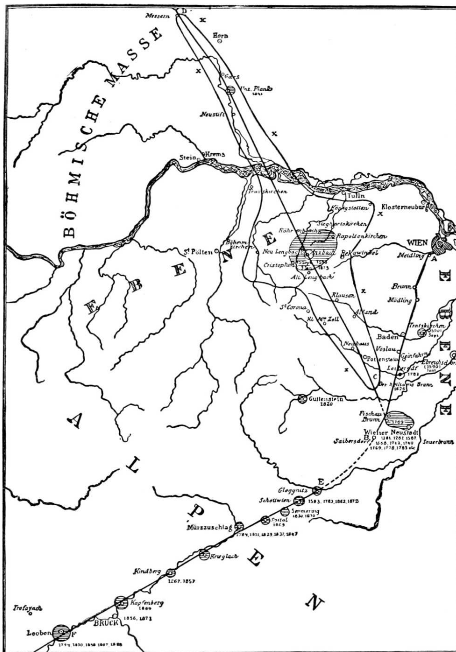
13: Fig. 13. — Jordbäfningslinjer i Nedre Österrike.
