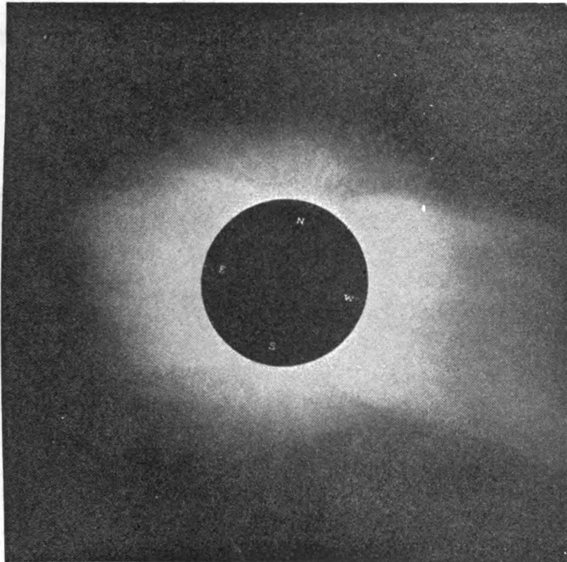
25: Fig. 25. — Fotografi av solkronan år 1900, motsvarande koronans utseende under minimiår av solfläckar. (Langley och Abbot.)
