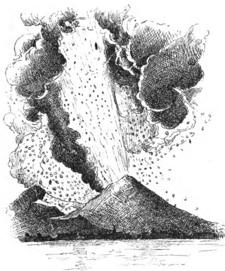
2: Fig. 2. — Vesuvii utbrott år 1794; efter en samtida handteckning.
