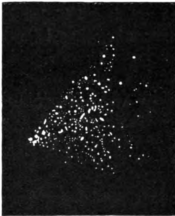
45: Fig. 45. — Kilformig stjärnhop i stjärnbilden Tvillingarne.
