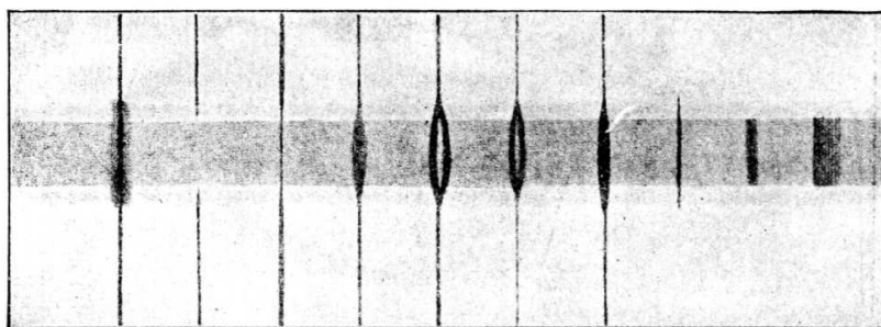
23: Fig. 23. — Schematisk bild av skillnaden mellan spektrum av en solfläck och det av den omgivande fotosfären enl. Mitchell. Några linjer synas i solspektrum av fotosfären men ej i fläcken, andra tvärtom, längst till höger två band. I midten två »omvända» linjer.
