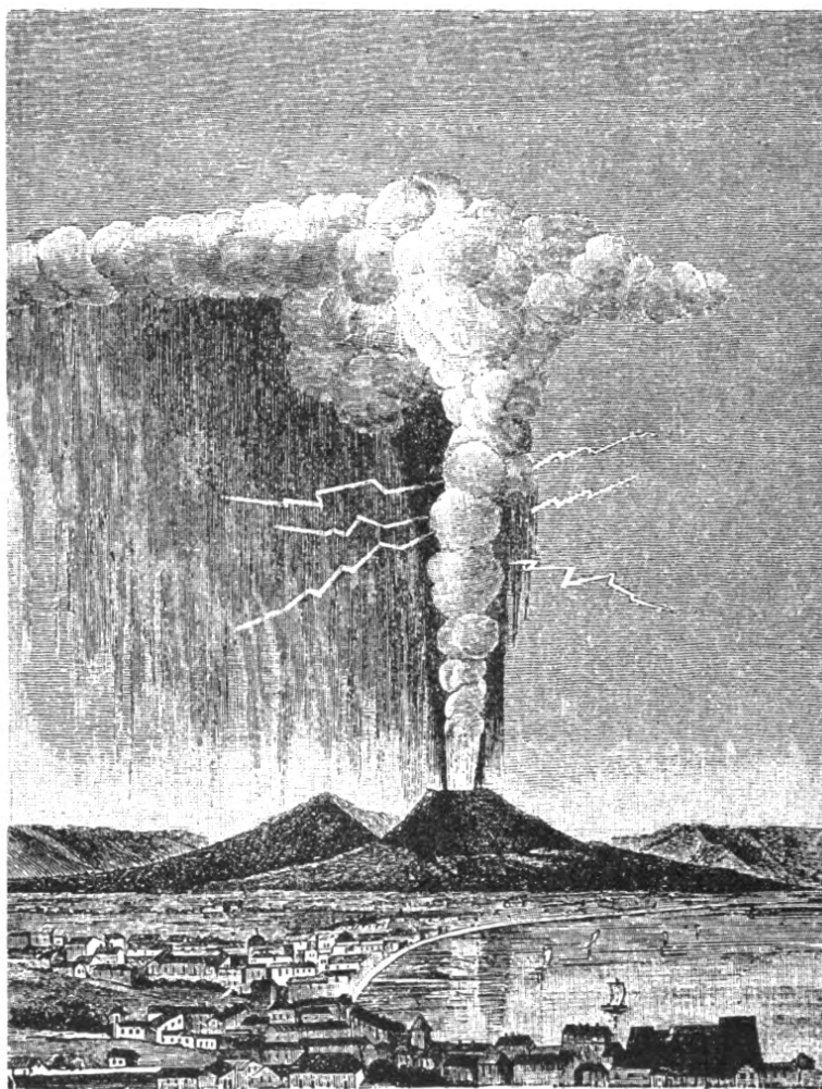
3: Fig. 3. — Vesuvii utbrott år 1822 efter en samtida handteckning.
