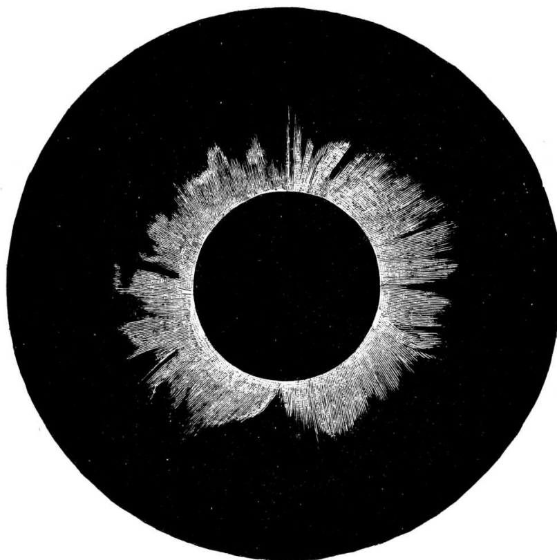
26: Fig. 26. — Fotografi av solkronan år 1870, tagen av Davis. 1870 var ett maximiår av solfläckar.
