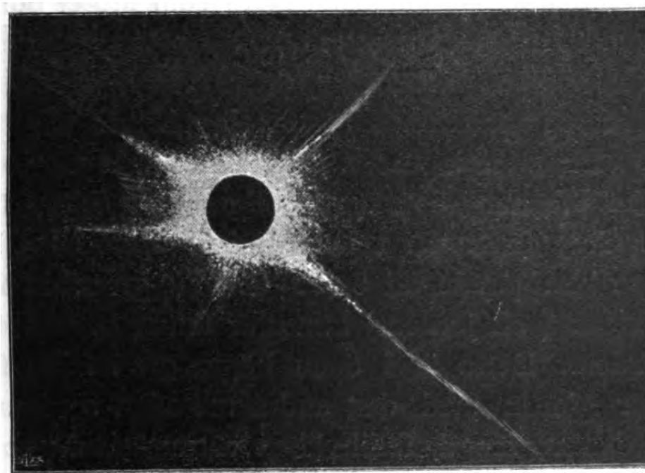
27: Fig. 27. — Fotografi av solkoronan år 1898 efter Maunder. 1898 var ett år med medelmåttigt antal solfläckar.
