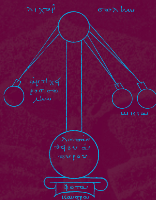
15 – Alambic à trois récipients (tribikos). Réduction aux 2/3.
