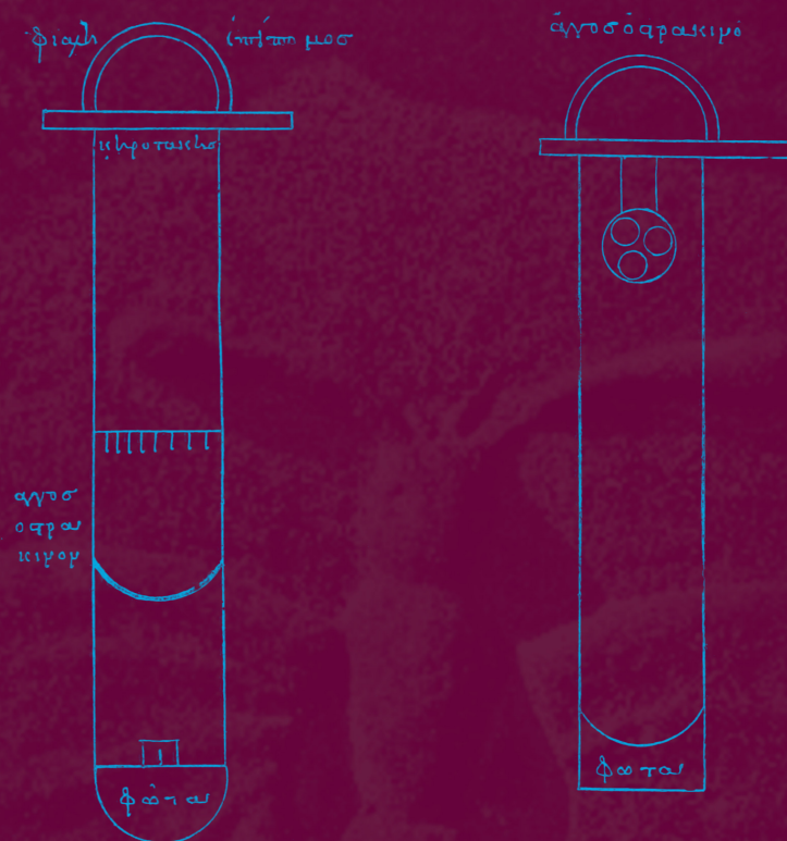
20 – Vases à digestion cylindriques. – Réduction aux \frac{2}{3} .
