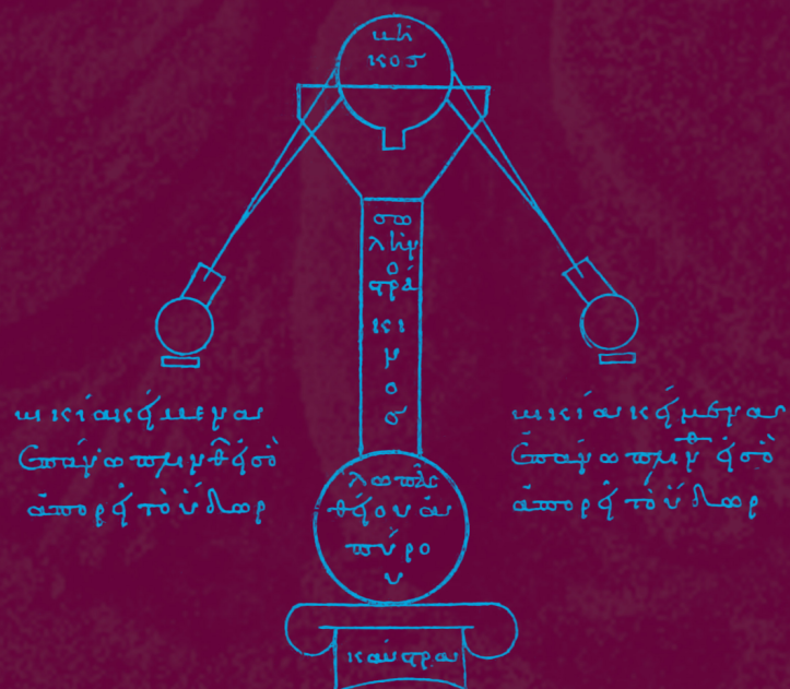
14 – Alambic à deux réceptifs (dibicos). Réduction aux 2/3.
