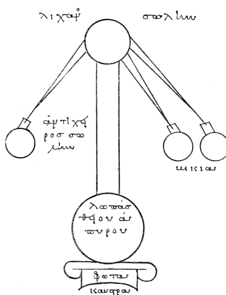
15 – Alambic à trois récipients ( tribicos ). Réduction aux 2/3.
