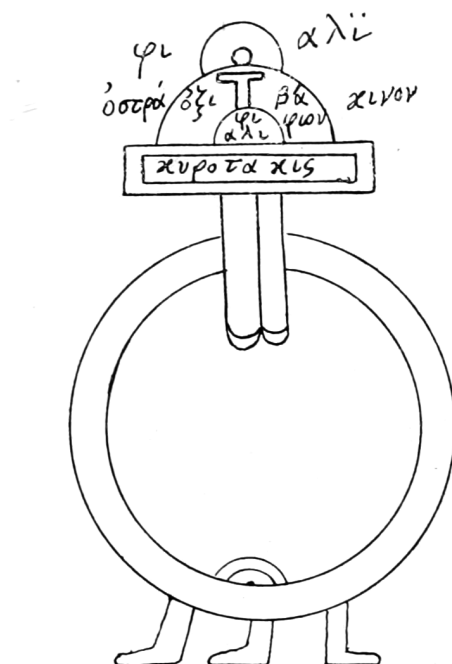
25 – Vase à kérotakis. — Décalque. Les inscriptions sont reproduites ici en caractères actuels, mais avec l'orthographe du manuscrit. — Réduction aux 2/3.
